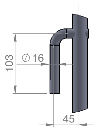
SECTION B SCALE 1 : 4
